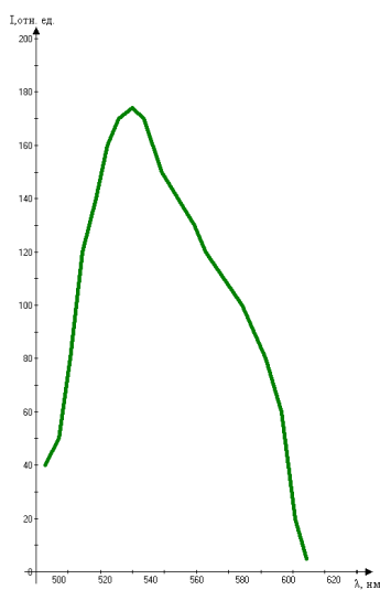
Fig. 2. Spectrul fotoluminescenței nanoparticulelor CdS în matrița polimerică a SEVILENului.
